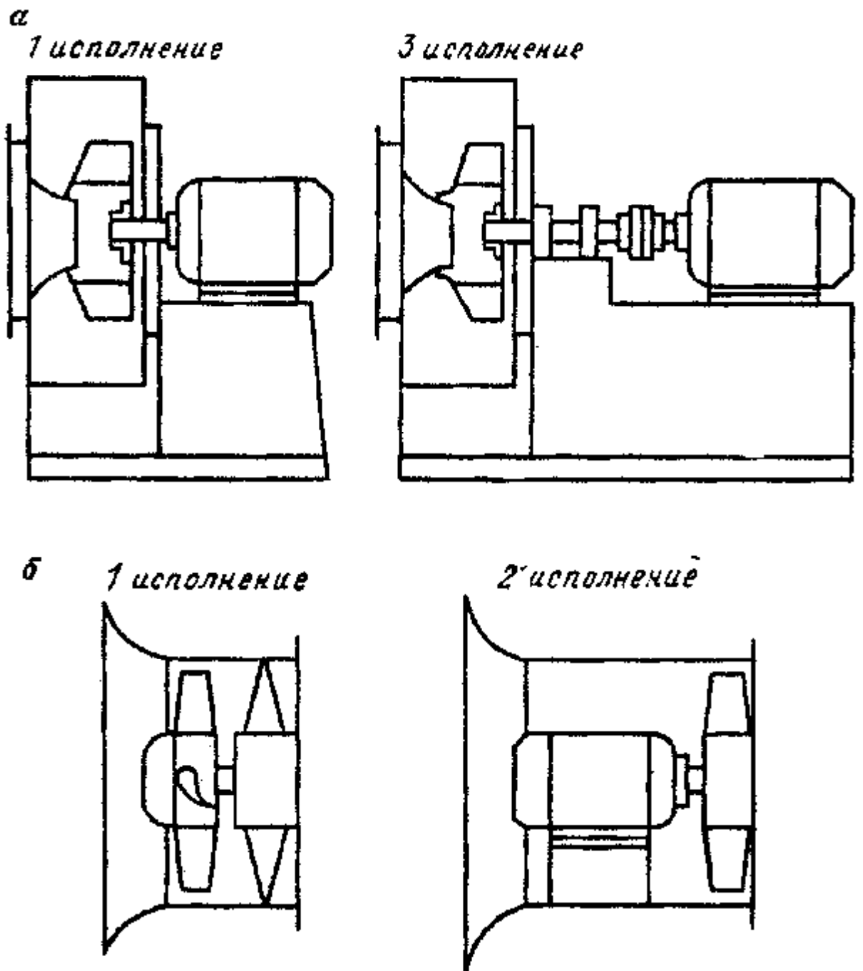
Рис. 1. Схемы конструктивных исполнений вентиляторов: а - радиальных; б - осевых
