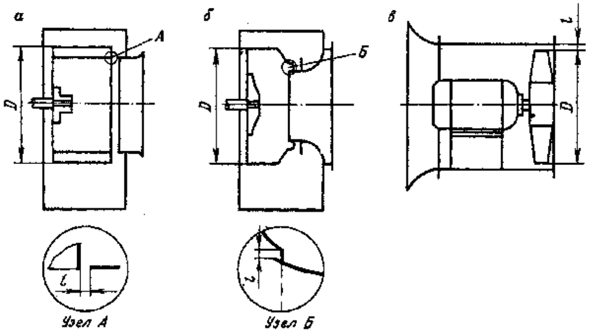
Рис. 2. Схемы зазоров вентиляторов: а - радиальных типа В.Ц14-46; б - радиальных типа В.Ц4-70; в - осевых ( l = 0,5-1,0 \%D )
