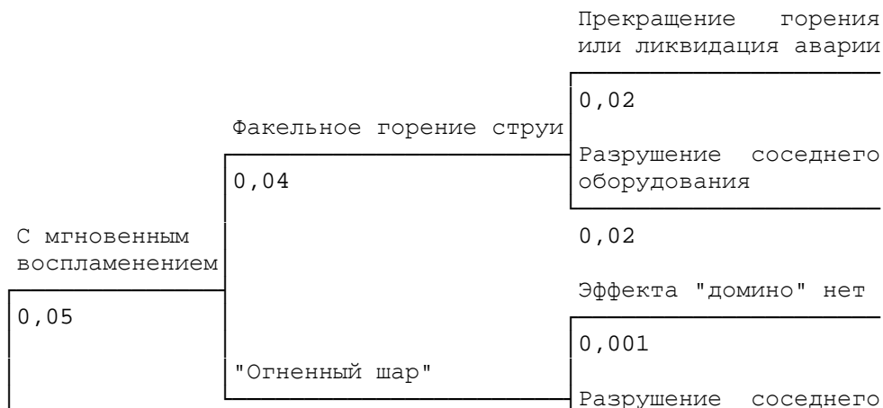
Рис. 1. "Дерево событий" аварий на установке первичной переработки нефти
