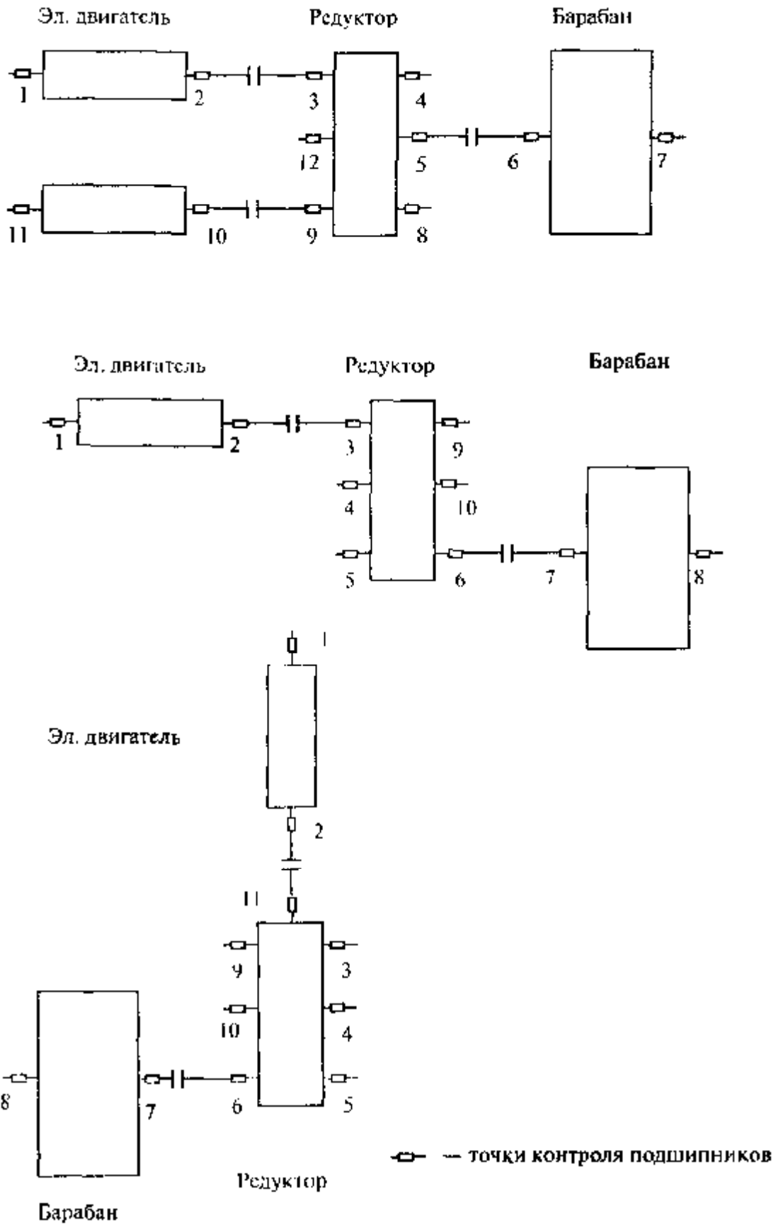
Рис. 1. Схема контроля вибрации
