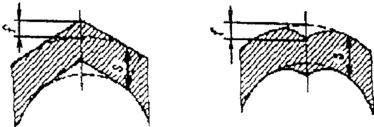
Рис. 1. Увод (угловатость) кромок в сварных швах
