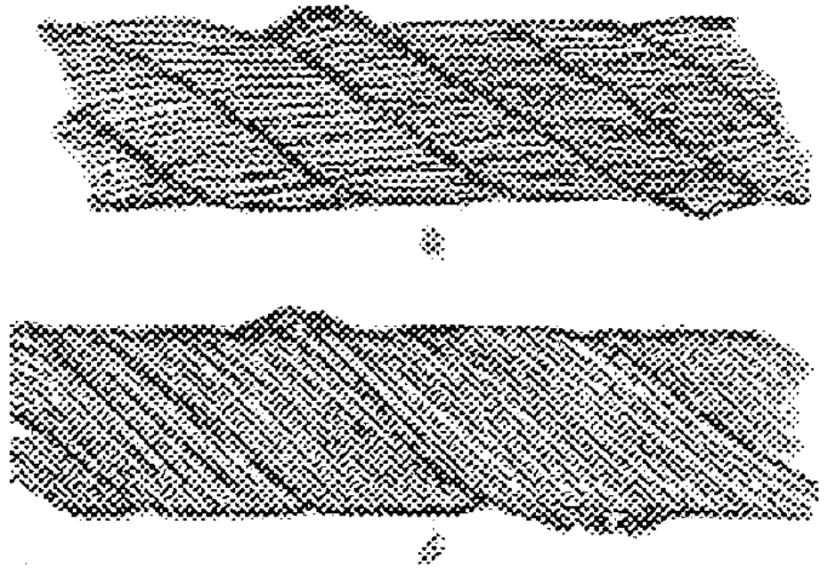
Рис. 2. Сочетание обрывов проволок с их износом: a - в канате крестовой свивки, б — в канате односторонней свивки
