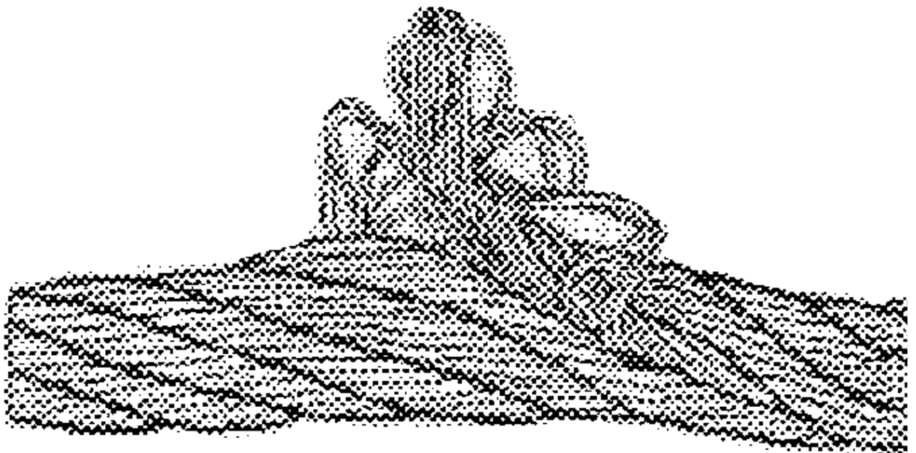
Рис. 11. Выдавливание сердечника
