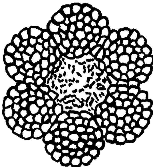
Рис. 8. Уменьшение площади поперечного сечения: проволоч (интенсивная внутренняя коррозия)
