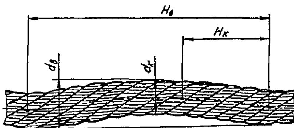
Рис. 9. Волнистость каната (объяснение в тексте)
