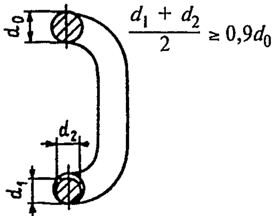
Рис. 2. Уменьшение диаметра сечения звена цепи:
