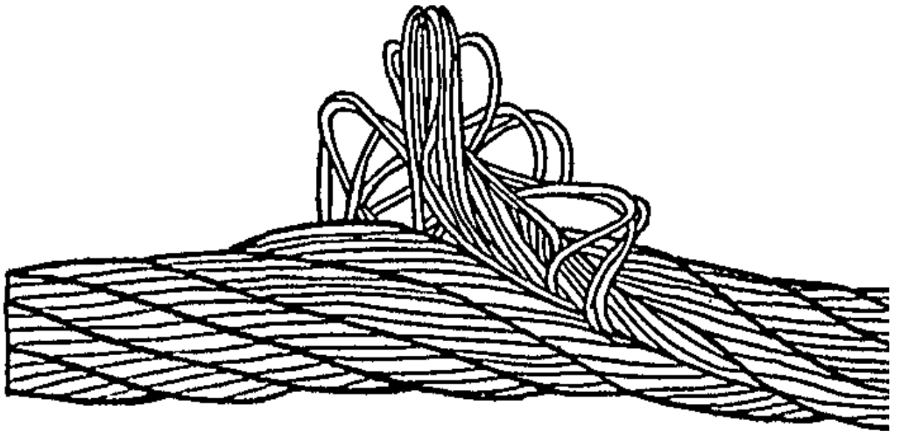
Рис. 11. Выдавливание сердечника
