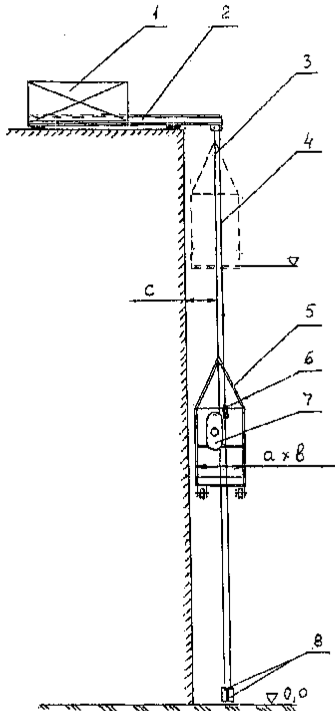
Пример чертежа общего вида
