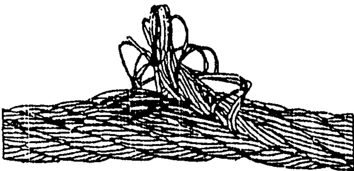
Рис.4. Выдавливание сердечника
