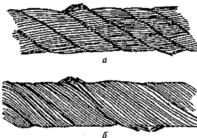
Рис. 2. Сочетание обрывов проволок с их износом:
