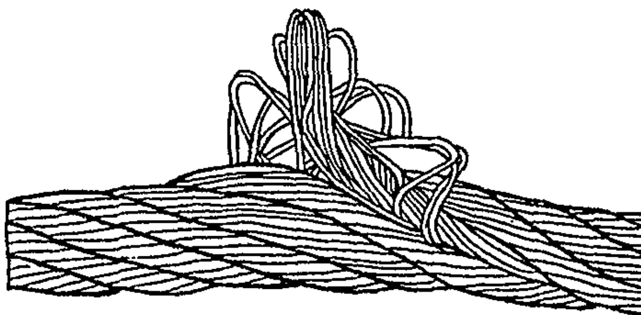
Рис. 10. Выдавливание сердечника
