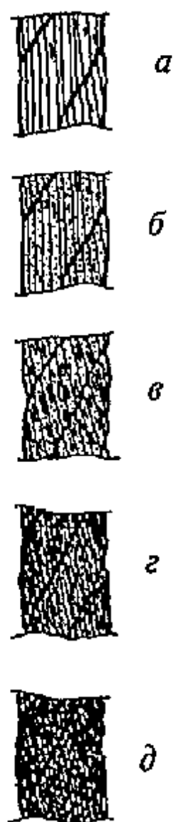
Рис. 5. Поверхностная коррозия проволок каната крестовой свивки:
