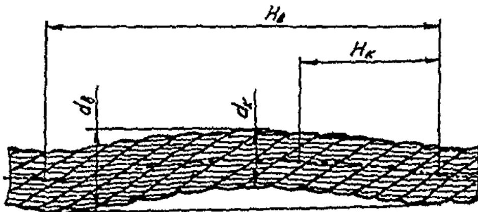
Рис. 8. Волнистость каната (объяснение в тексте)
