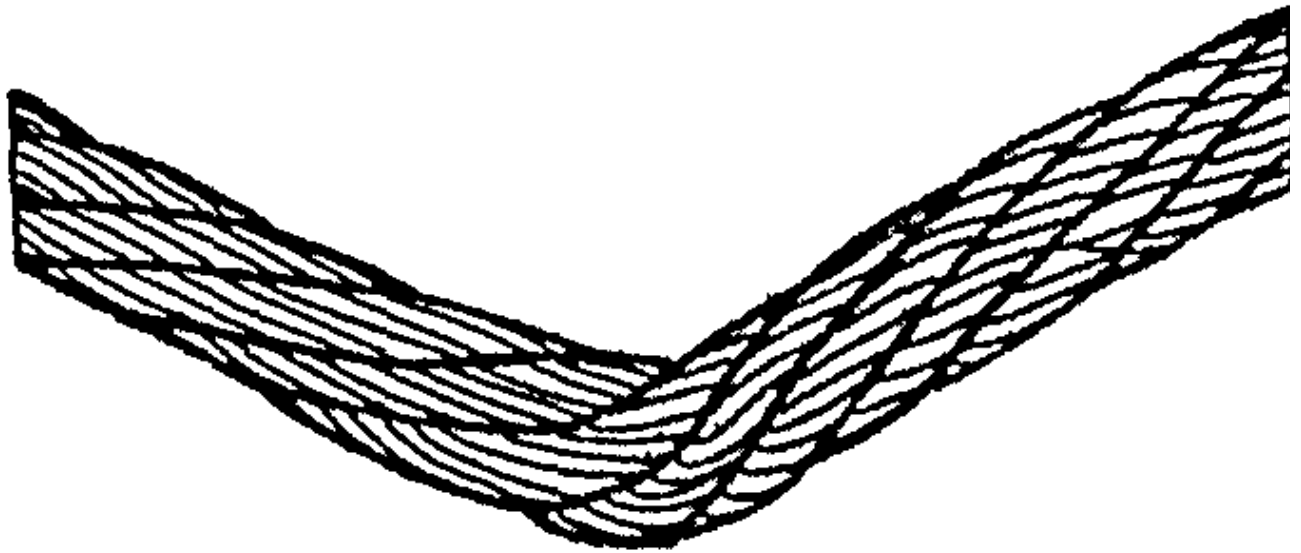
Рис. 16. Перегиб каната
