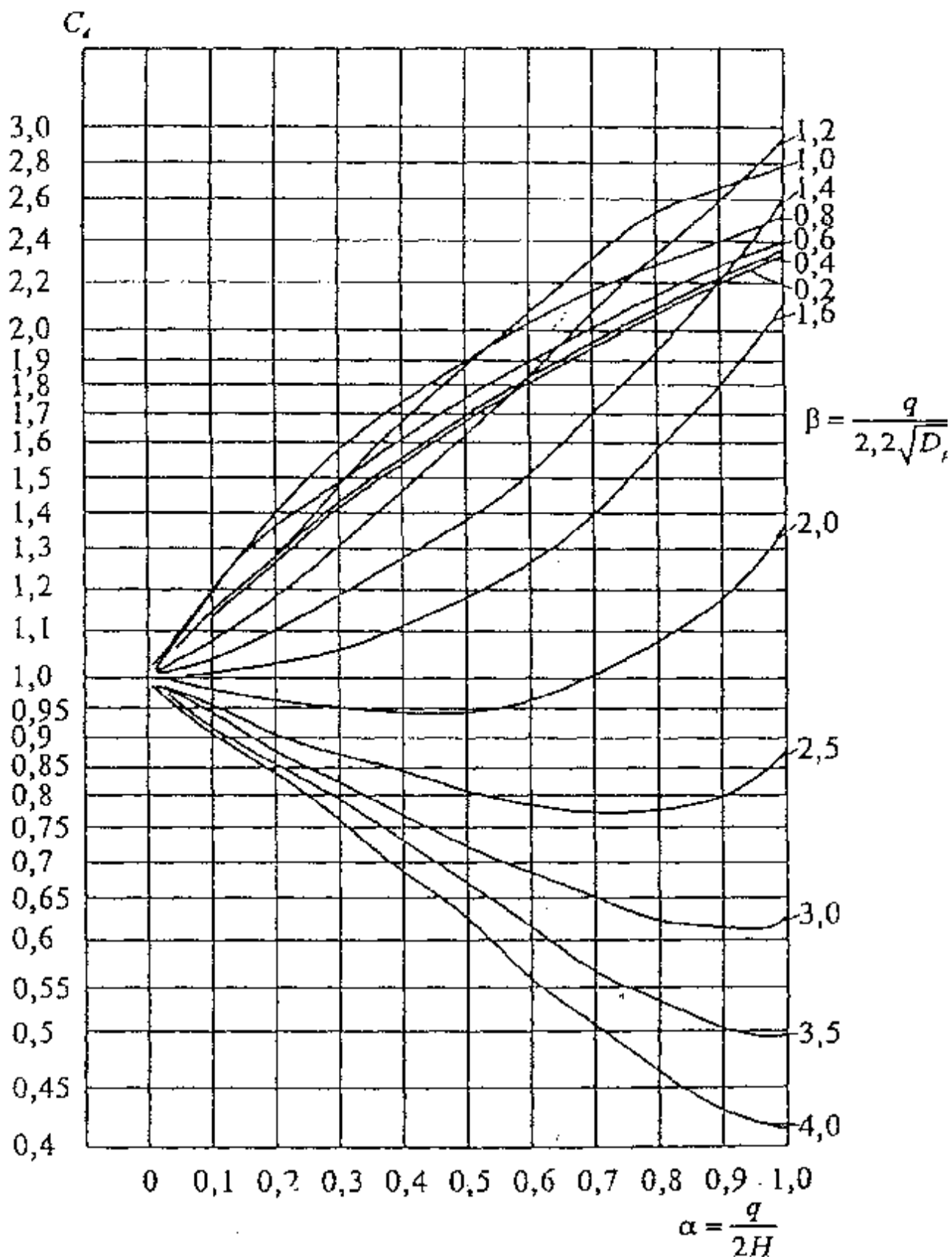
Рис. 5.10. Графики для определения коэффициента C_s
