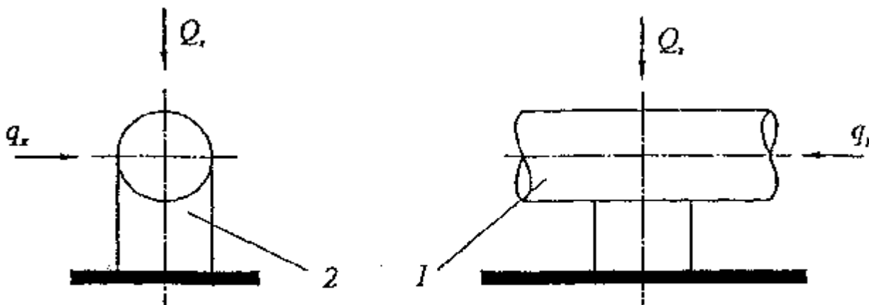
Рис. 5.1. Схема нагрузок на опору: 1 — труба; 2 — подвижная опора
