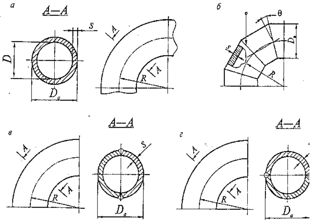
Рис. 4.1. Отводы: а — гнутый; б — секторный; в, г — штамповарной
