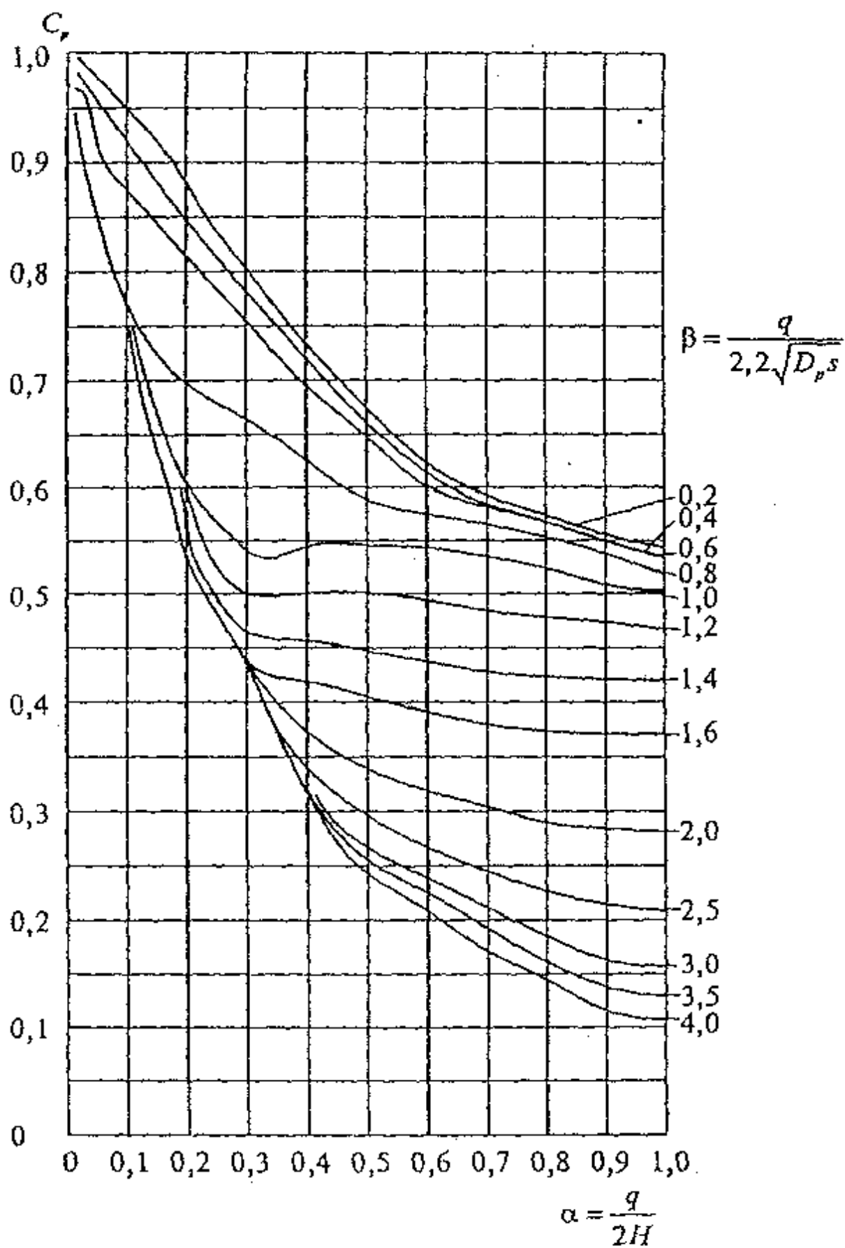
Рис. 5.9. Графики для определения коэффициента C_r
