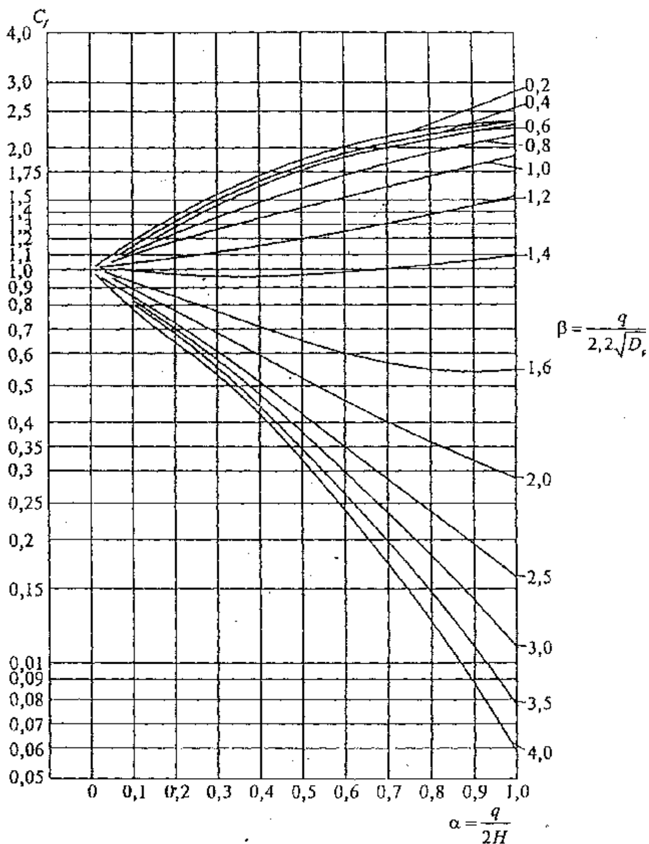
Рис. 5.8. Графики для определения коэффициента C_f
