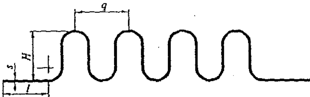
Рис. 5.5. Гибкий элемент компенсатора
