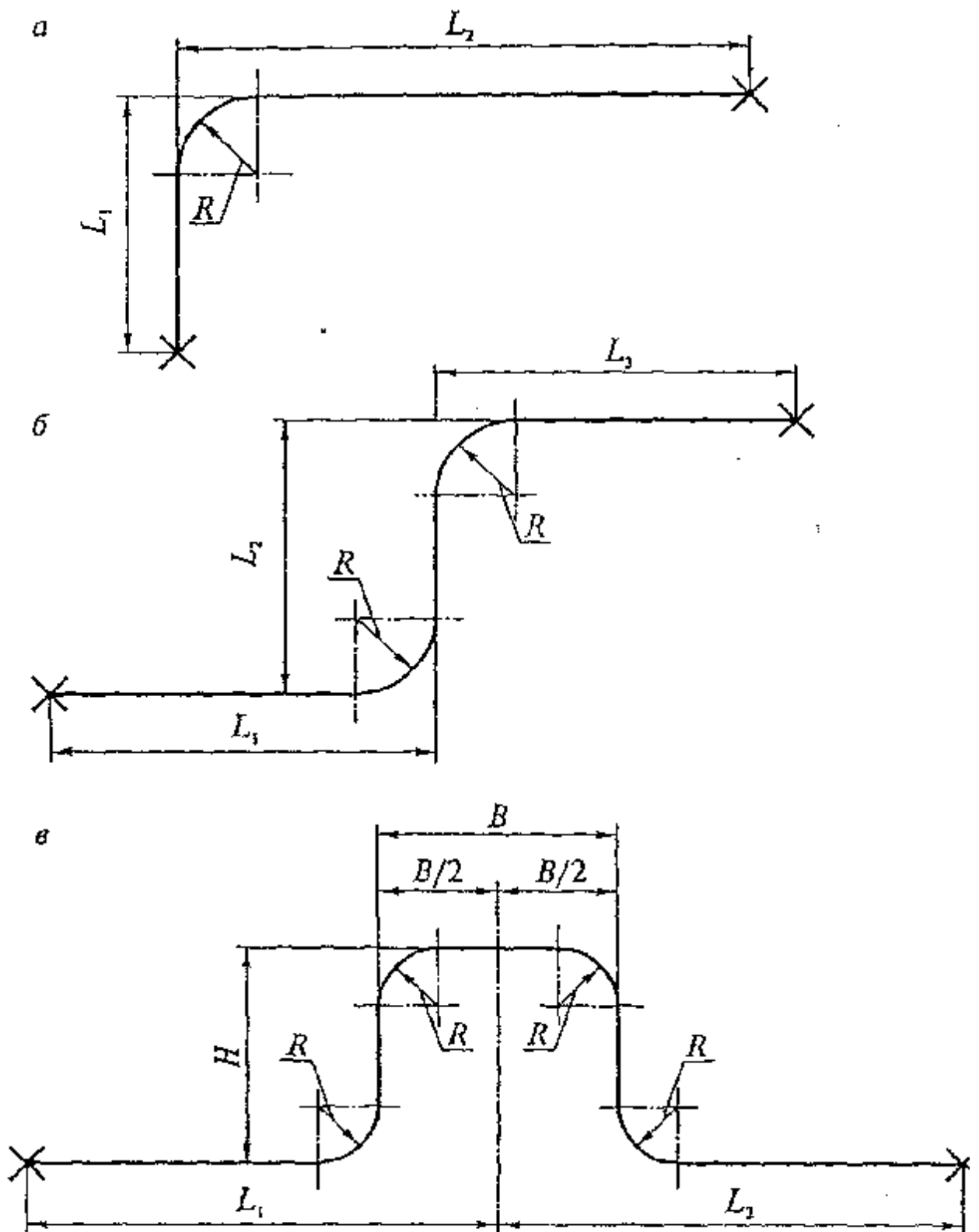
Рис. п. 3.1. Схемы участков трубопроводов с прямыми углами: a — Г-образной формы; b — Z-образной формы; c — П-образной формы
