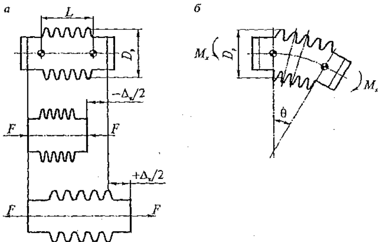
Рис. 5.6. Схема работы компенсатора: а — осевого; б — углового
