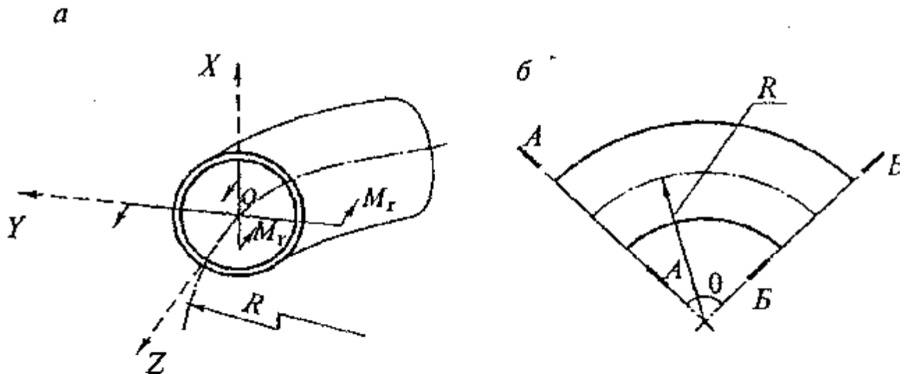
Рис. 5.3. Расчетная схема отвода: а — схема нагружения; б — расчетные сечения
